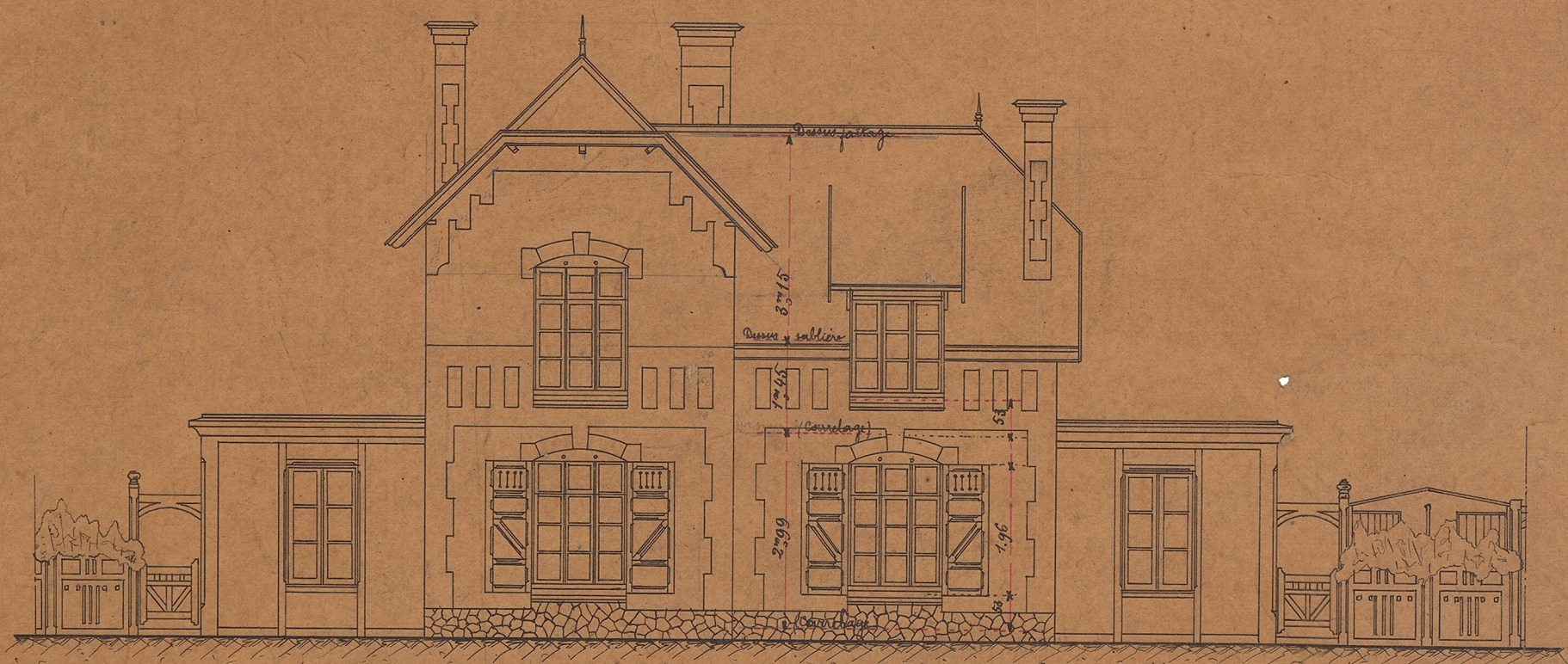
ELEVATION
