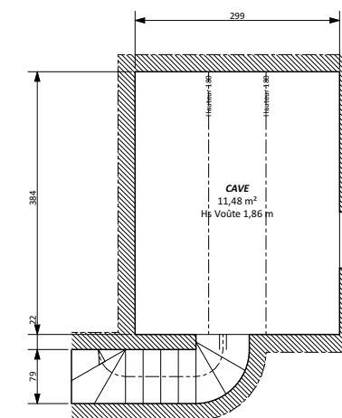
Plan Sous-sol
