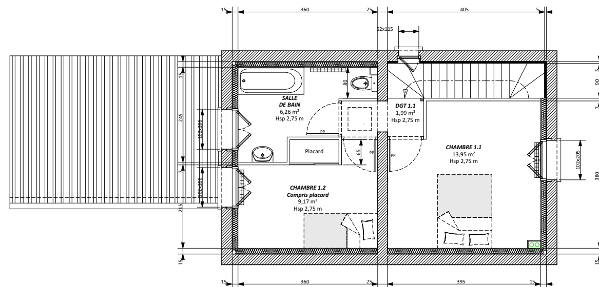
Plan Etage
