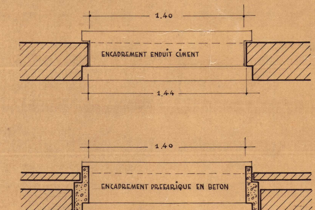
VARIANTE D'ENCADREMENT DES BAIES ECHELLE 0.05 P.M.
