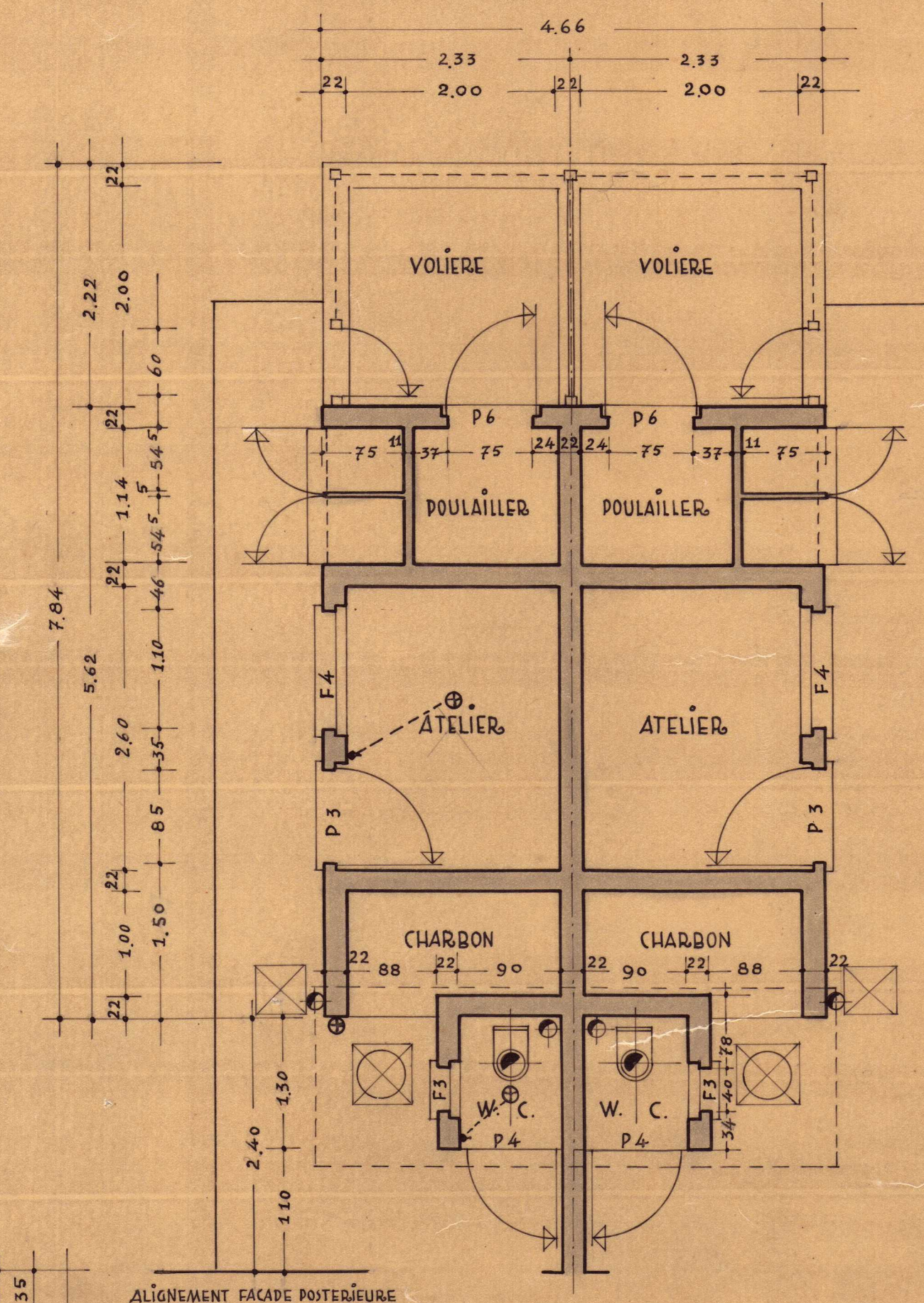
VARIANTE DEPENDANCES POUR TYPE AVEC CAVE
