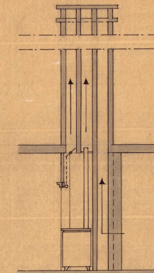
DETAIL DES CHEMINÉES
