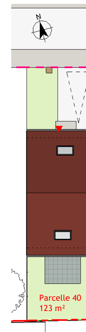
Plan de masse Logt 40 Ech : 1 : 200
