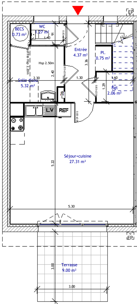
REZ DE CHAUSSEE - Logt 40 Ech : 1 : 100
