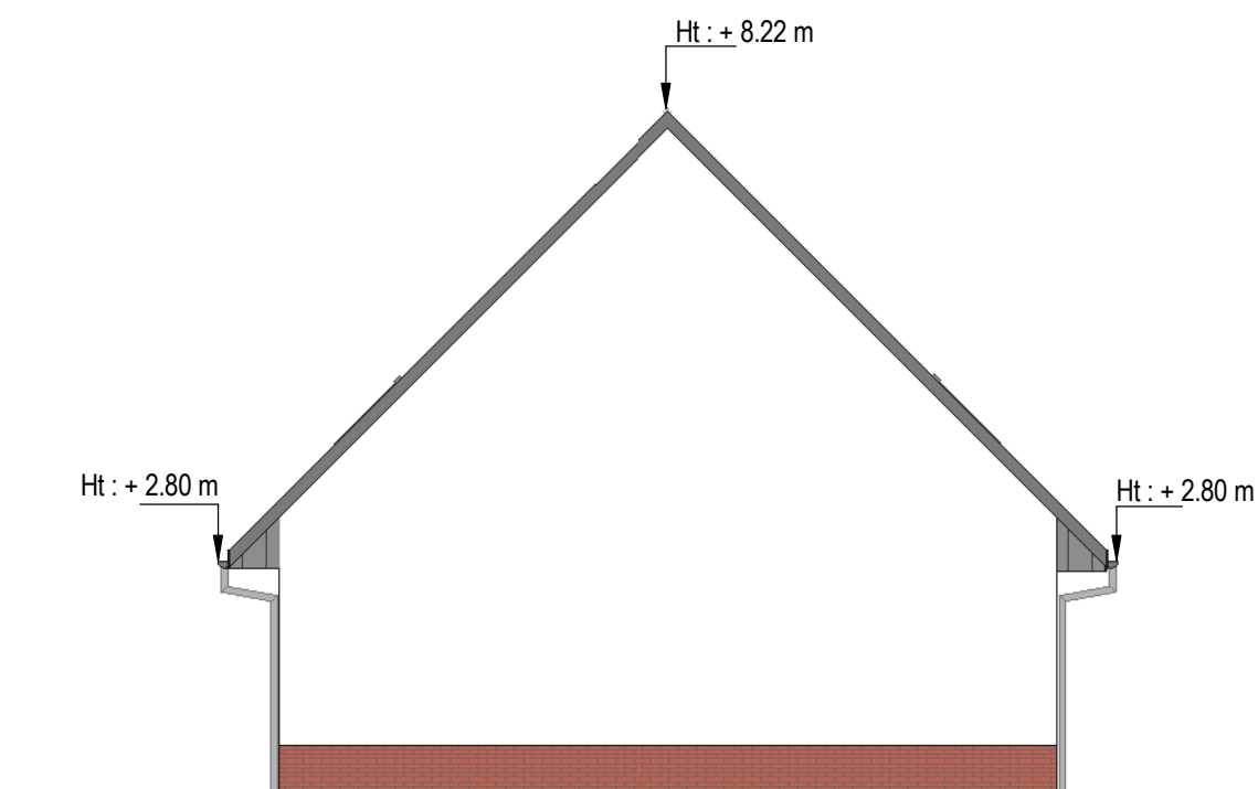
Pignon Ouest Logt 40
