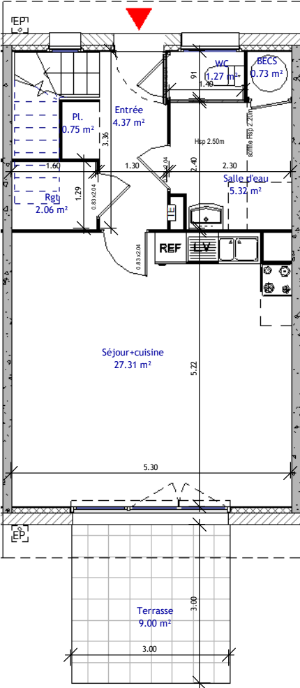
REZ DE CHAUSSEE - Logt 38 Ech : 1 : 100
