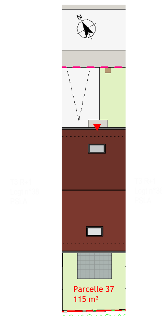
Plan de masse Logt 37 Ech : 1 : 200
