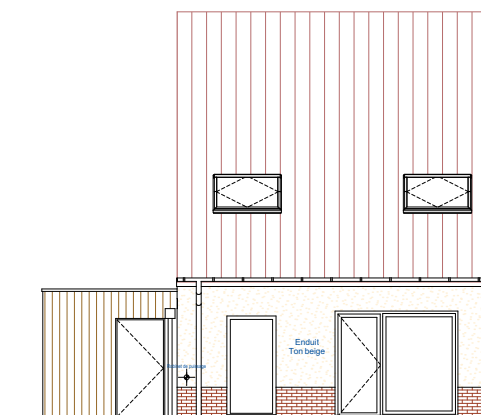
Façade Jardin
