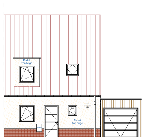
Façade Rue
