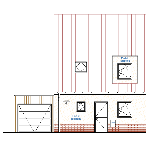
Façade Rue
