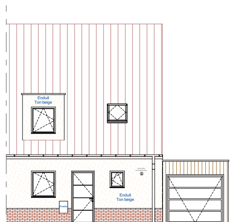
Façade Rue
