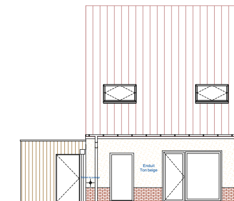
Façade Jardin
