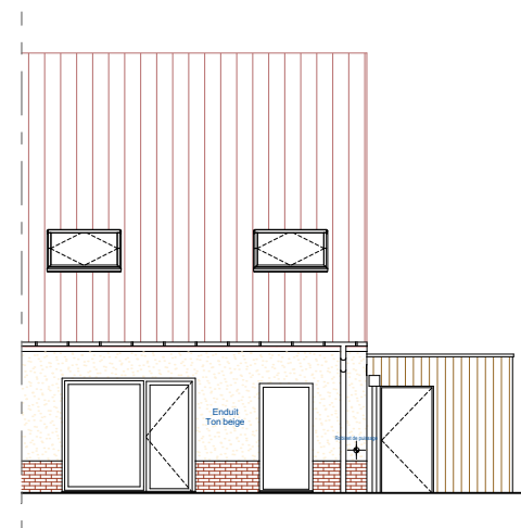
Façade Jardin
