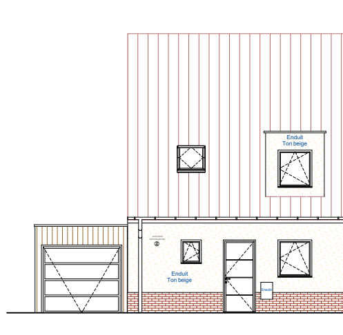
Façade Rue
