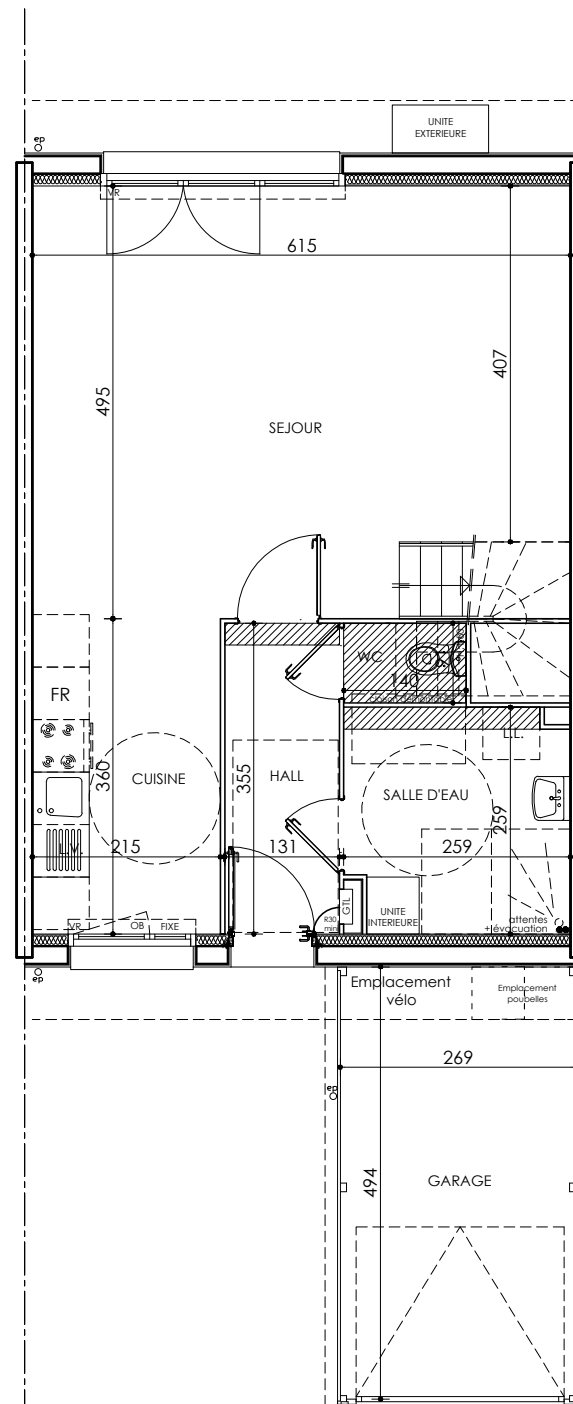
Rez-de-Chaussée
